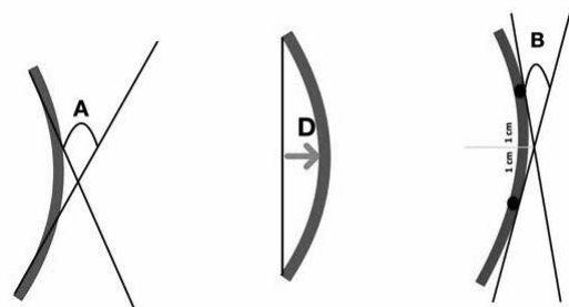
A: Rod end angle B: Rod apex angle D: Rod deflection
